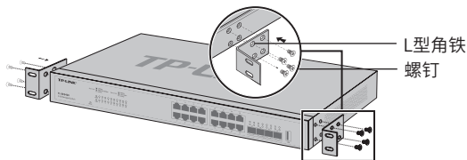
图2-2 角铁安装示意图
