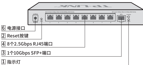
图1-5 TL-SE2109后面板示意图
