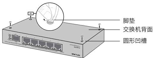
图2-1 桌面安装示意图
