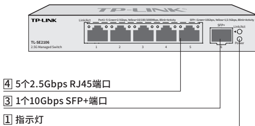
图1-2 TL-SE2106前面板示意图
