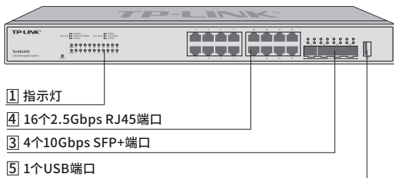
图1-7 TL-SE2420前面板示意图
